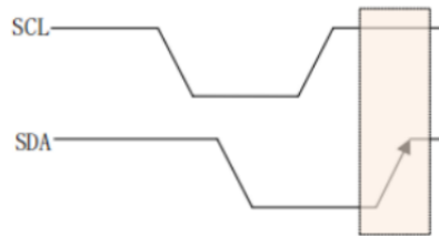
图 9-6 I2C 终止信号
